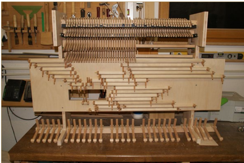
Koppelchassis vor Einbau der Abzugsdrähte
